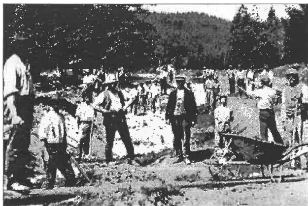
Výkop pro plánovanou stavbu vodní elektrárny u původního mostku přes potok Orlička v dnešní Bublačce. Plánovanou stavbu vodní elektrárny o výkonu 220 HP (koňských sil) v důsledku pozdějšího zatopení údolí Divoké Orlice p. Josef Wagner z Pastvín č.p.30 již nedokončil.
